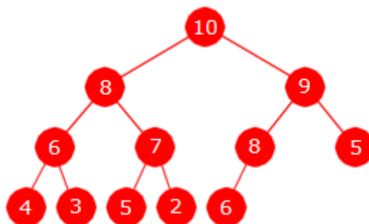
Figur 1.2.11.d : En maksimumsheap
